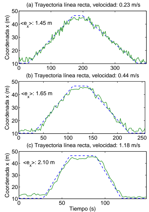
Figura 11: Desplazamiento entre los puntos A y B del edificio (ver figura 6) a tres velocidades distintas, y error medio en la posición lineal ( e_x = \hat{x} - x ).
