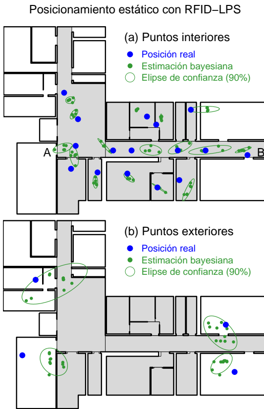
Figura 6: Localización en puntos estáticos con el sistema RFID-LPS: (a) puntos interiores al área sombreada donde están colocados los marcadores RFID (475 m 2 ); (b) puntos exteriores a dicha área. Las dimensiones máximas del edificio son 45.40×32.40 m, y su área total de 910 m 2 .
