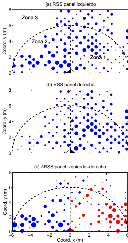
Figura 12: Medidas experimentales de fuerza de señal del sensor con dos antenas de panel, con orientación relativa de 90°. (a) y (b) RSS individuales medidas por los paneles izquierdo y derecho; (c) diferencia \Delta RSS (diámetro de los círculos proporcional a |\Delta RSS); color azul si \Delta RSS > 0 y rojo en caso contrario.
